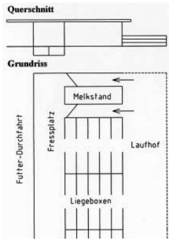
Stallskizze (Ausschnitt aus Grundriss und Querschnitt)
